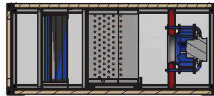
A-A ( 1 : 16 )
