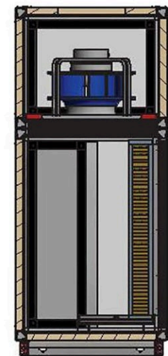
A-A (1 : 25)
