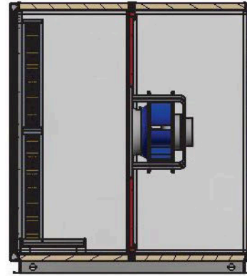
A-A ( 1 : 30 )
