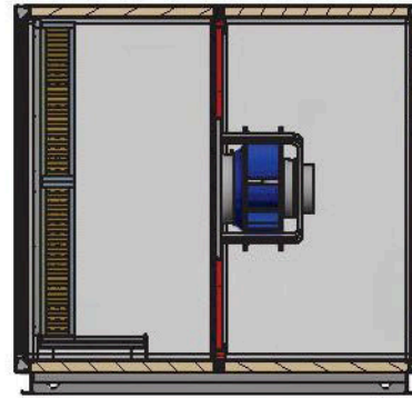
A-A (1 : 28)
