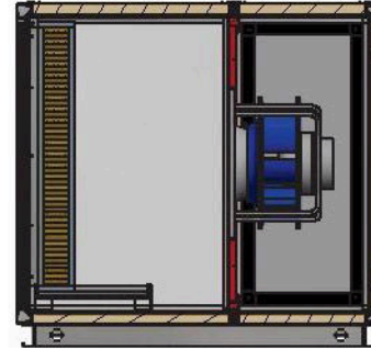
A-A (1 : 26)
